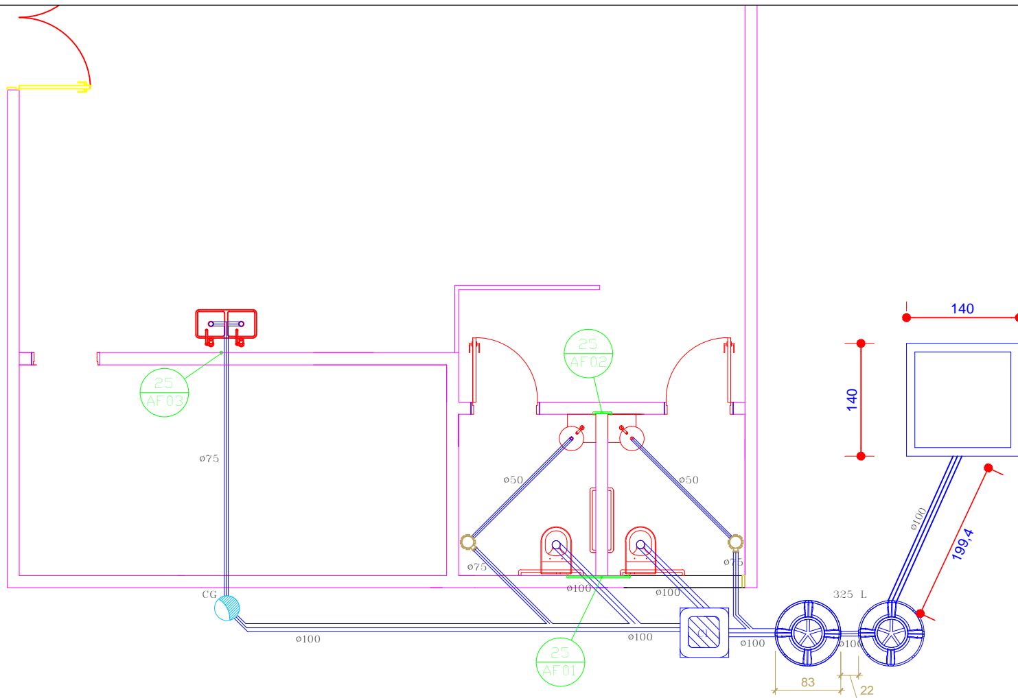
8 PLANTA BAIXA - HIDROSSANITÁRIO Escala: 1/100
