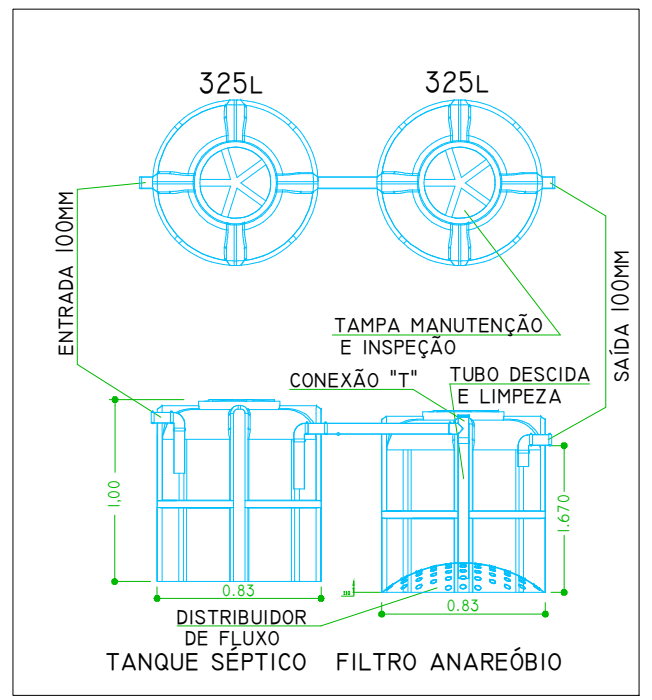
7 TANQUE SÉPTICO E FILTRO ANAREÓBIO SEM ESCALA
