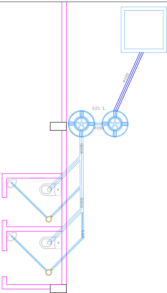
5 HIDROSSANITÁRIO Sem Escala
