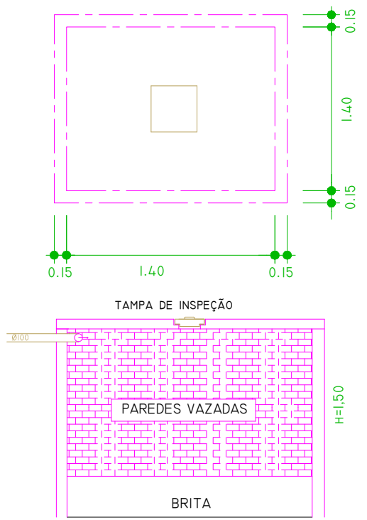
6 POÇO SUMIDOURO SEM ESCALA
