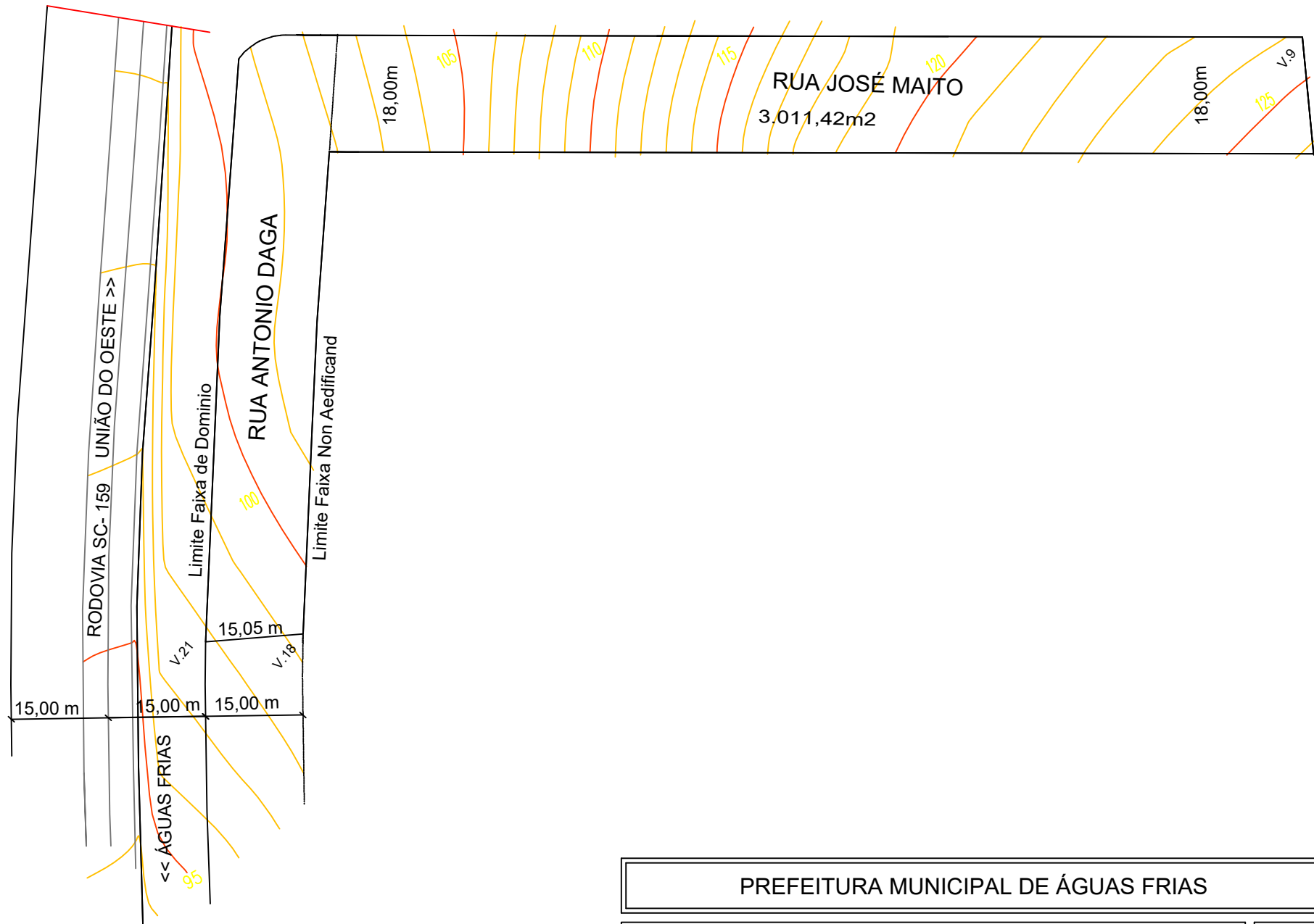
3 PLANIALTIMÉTRICO RUA - FONTE AMOSC Escala 1:500
