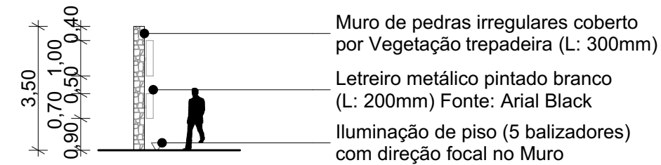
VISTA LATERAL
