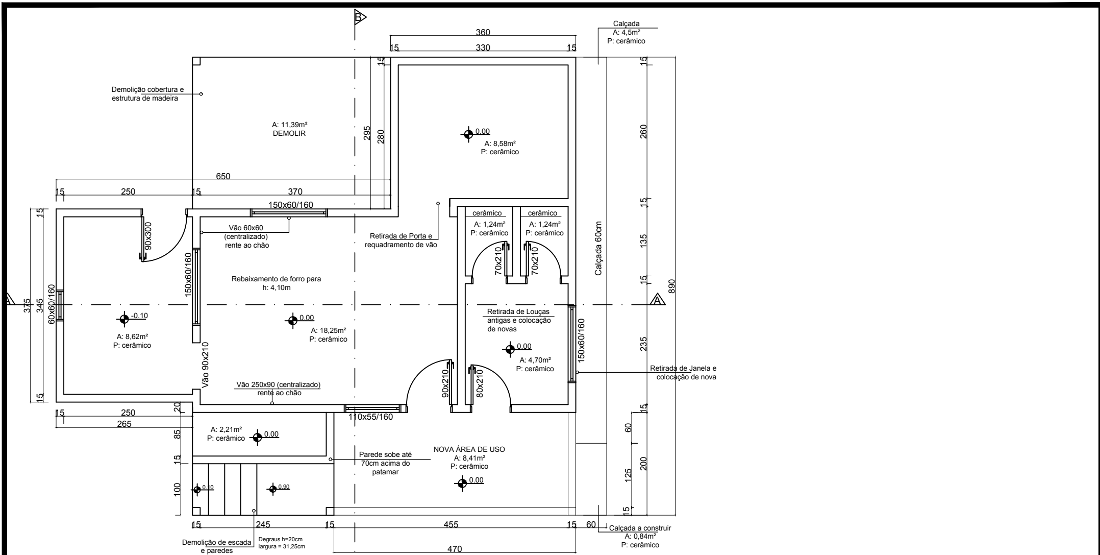
1 PLANTA BAIXA Escala: 1/75 Área: 64,85m 2
