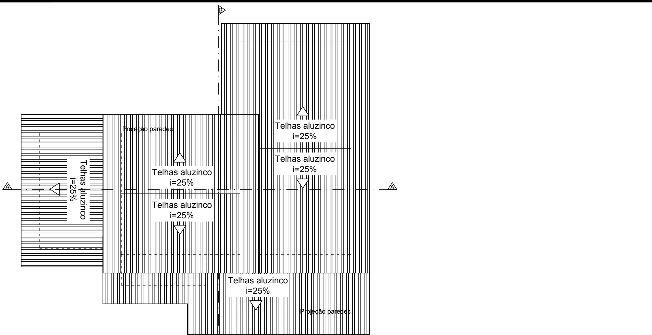
2 PLANTA DE COBERTURA Escala: 1/75
