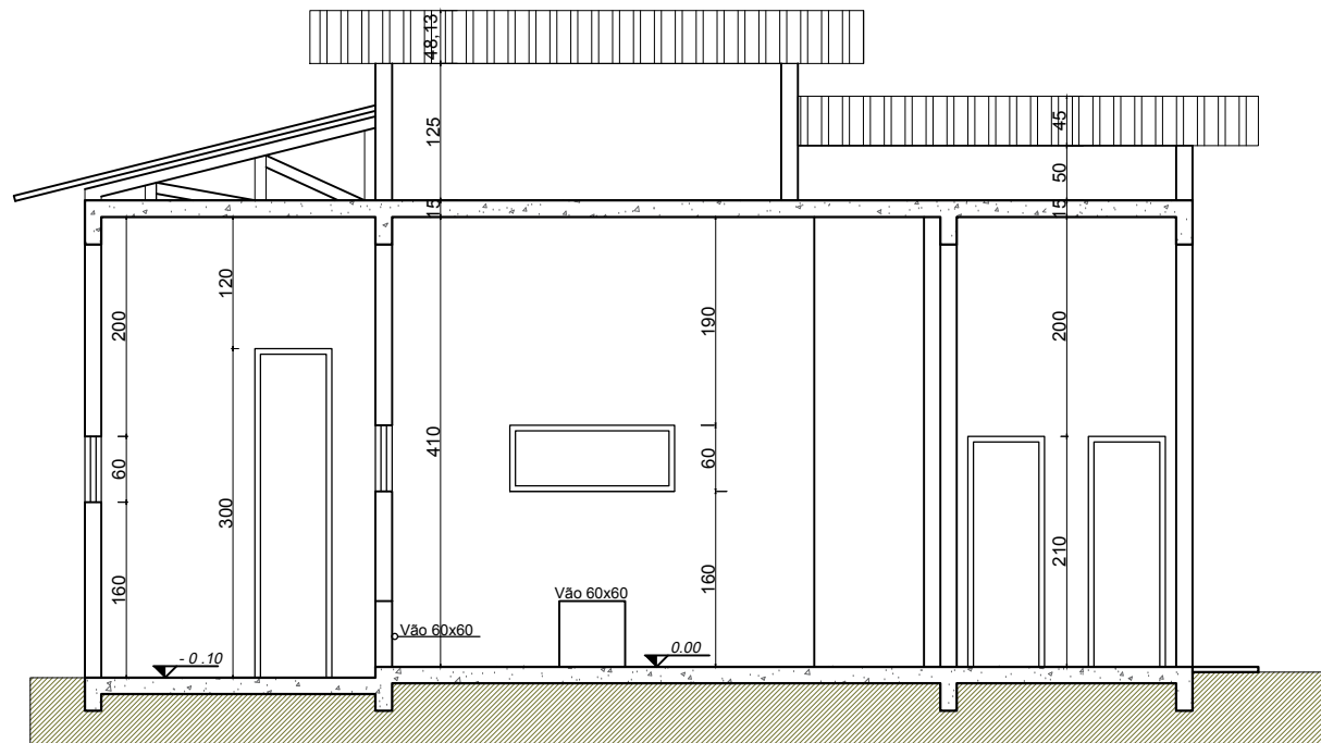
3 CORTE A-A Escala: 1/75
