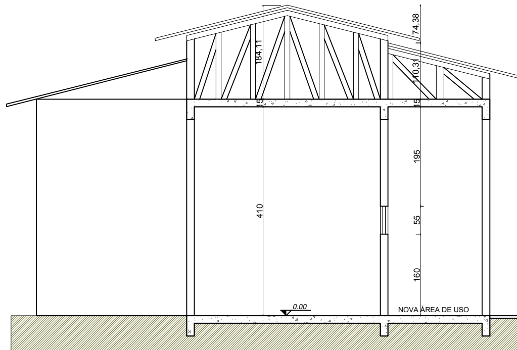
4 CORTE B-B Escala: 1/75
